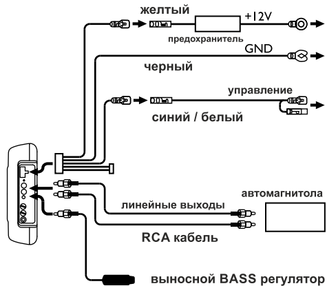
А. Схема подключения сабвуфера к головному устройству через НЧ линейные входы RCA
