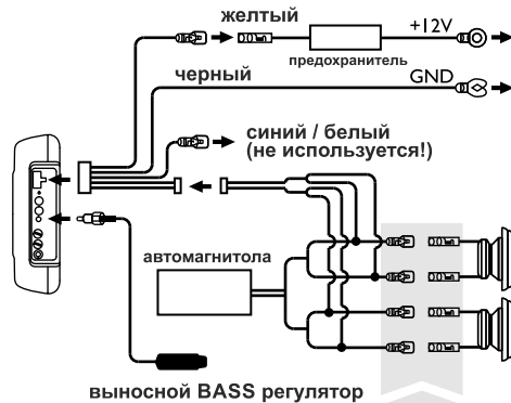
В. Схема подключения сабвуфера к головному устройству по высокоуровневым входам (к динамикам)
